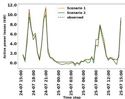
Slika 7.a: Faza A
