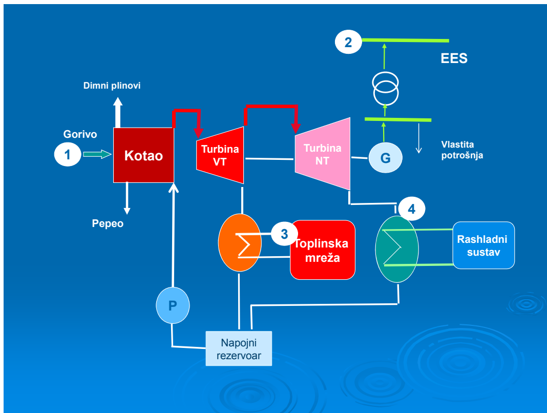
Slika 3. Osnovna shema kogeneracijskog bloka na vodenu paru P - napojna pumpa
